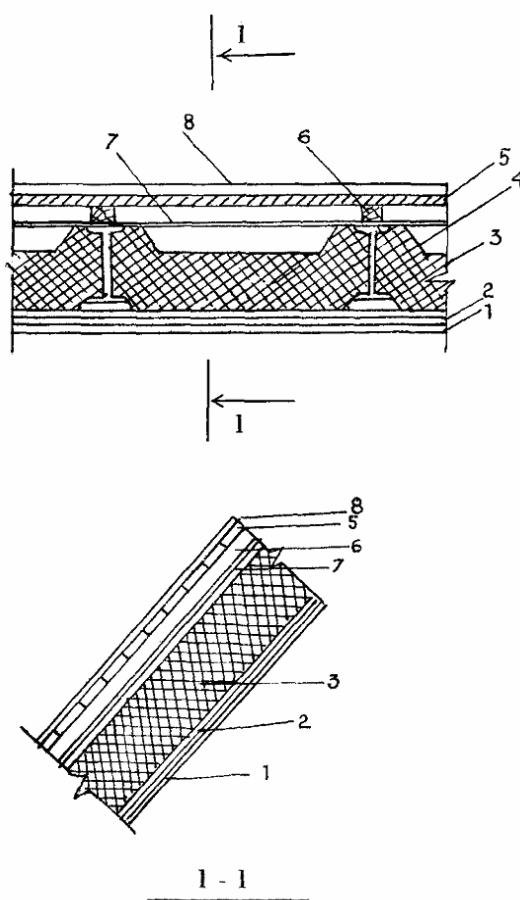
Рис. 8. Конструкция мансардной кровли с несущими металлическими конструкциями: 1 - подшивной потолок; 2 - пароизоляция; 3 - металлические стропила; 4 - утеплитель; 5 - диффузионная пленка; 6 - обрешетка; 7 - деревянные бруски; 8 - водоизоляционный ковер из плоских или профильных листов, цементно-песчаной черепицы
