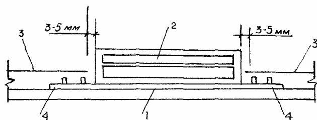
Рис. 13. Примыкание водоизоляционного ковра к мансардным окнам:
