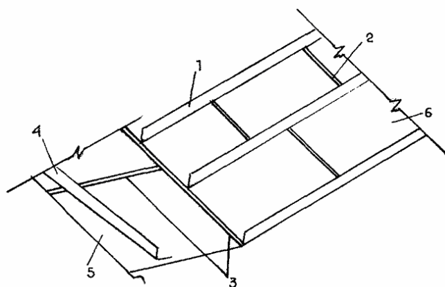
Рис. 11. Место сопряжения ската кровли с карнизом при организованном водостоке для водоизоляционного ковра из цинк-титана или меди:
