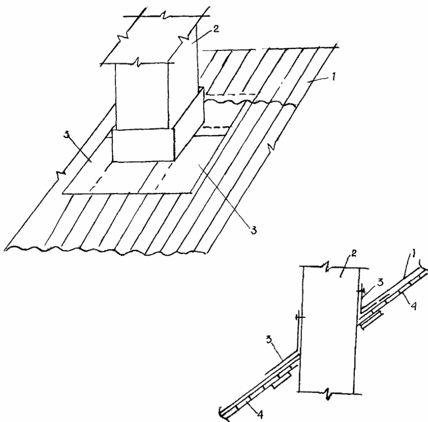
Рис. 14. Место примыкания водоизоляционного ковра к вентиляциям, дымоходам и т.п.:
