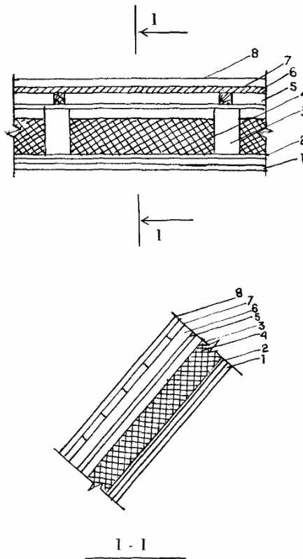
Рис. 7. Конструкция мансардной кровли с несущими деревянными конструкциями:
