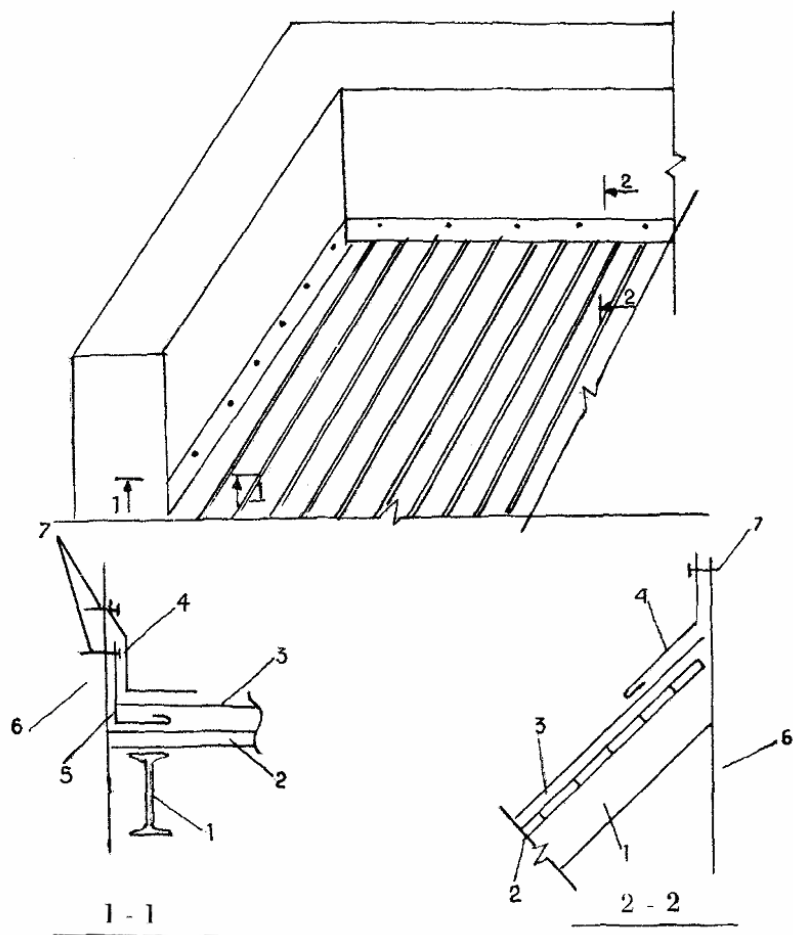
Рис. 12. Места примыкания к стенам и парапетам по уклону и горизонтали:
