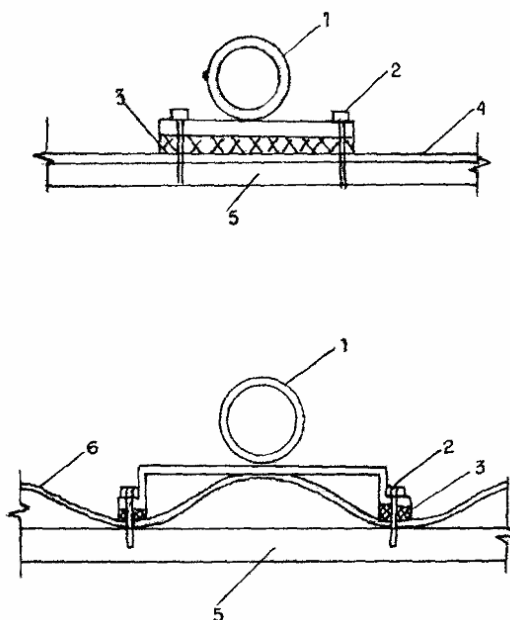
Рис. 16. Узлы крепления анкеров при различных материалах водоизоляционных ковров:
