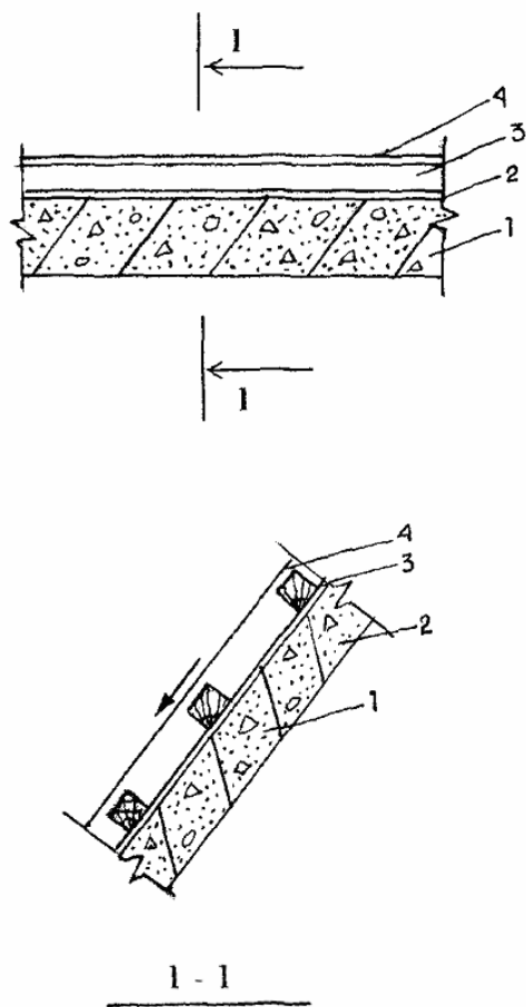
Рис. 5. Кровля с несущей железобетонной плитой:
