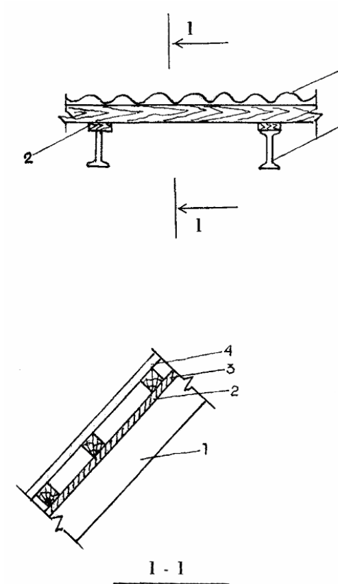
Рис. 4. Кровля с несущими металлическими конструкциями и водоизоляционным ковром из профилированных листов:
