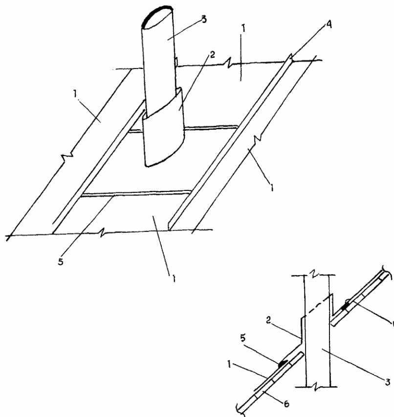
Рис. 15. Место примыкания водоизоляционного ковра к технологическим трубопроводам:
