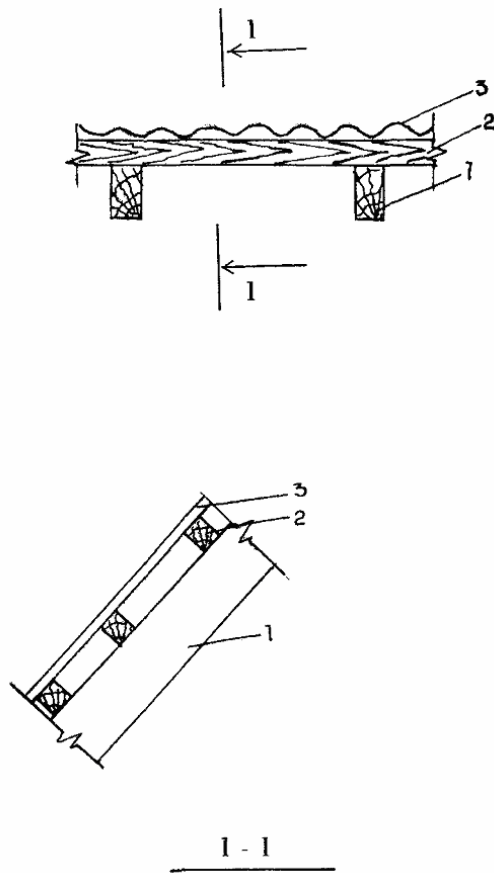
Рис. 3. Кровля с несущими деревянными конструкциями и водоизоляционным ковром из профильных листов:
