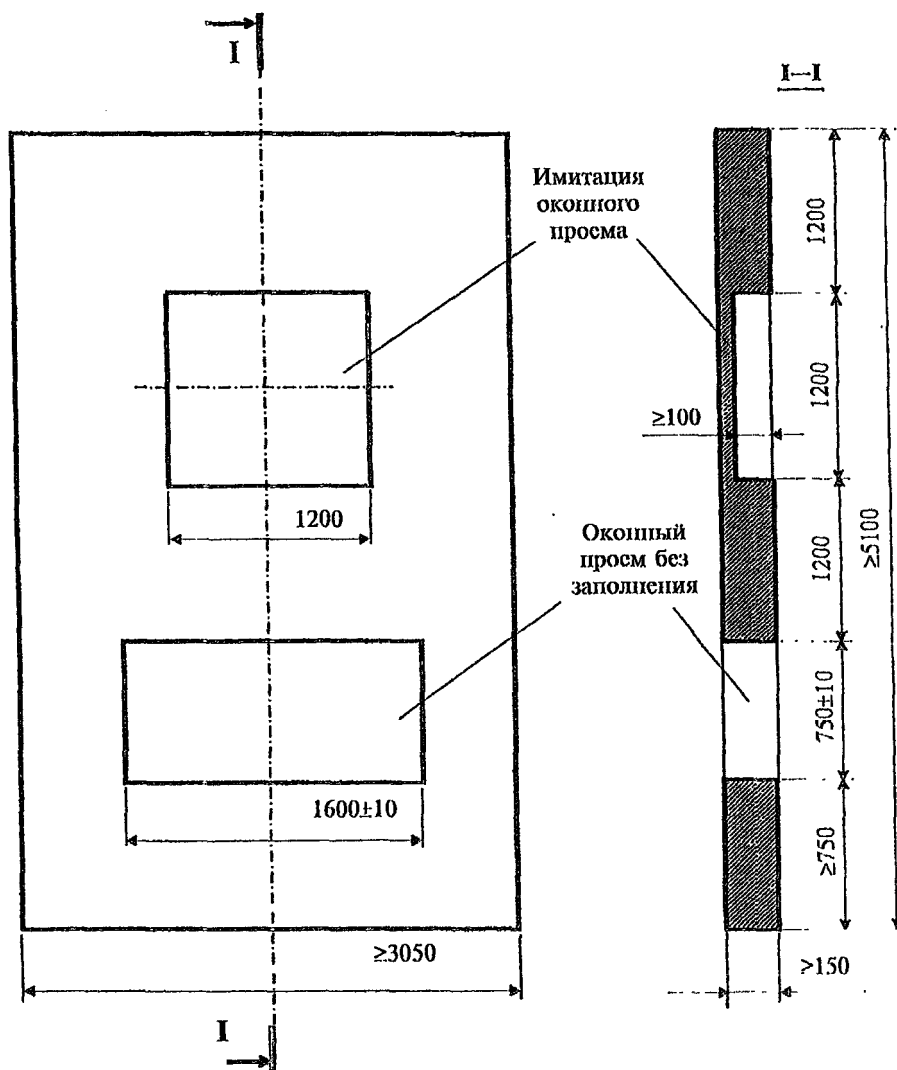
Рисунок 1. Фрагмент стены
