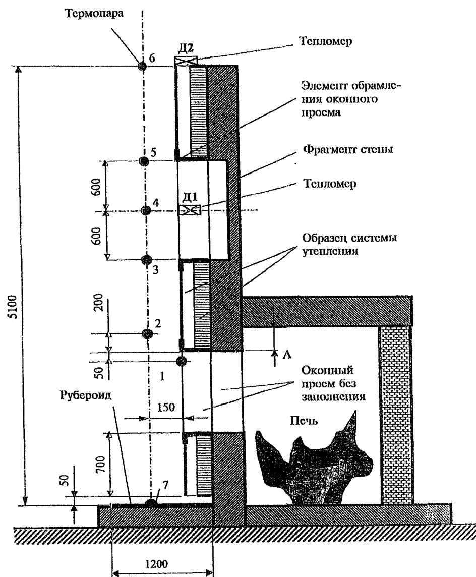
Рисунок 26. Схема установки с образцом системы утепления Разрез I - I
