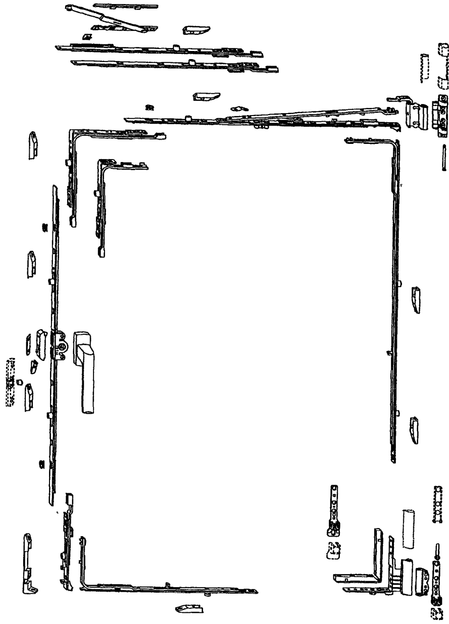
Рисунок Б.3. Устройство поворотнo-откиднoе
