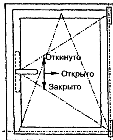
Рисунок А.3. Устройство поворотно-откидное
