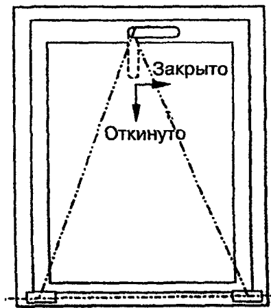
Рисунок А.2. Устройство откидное
