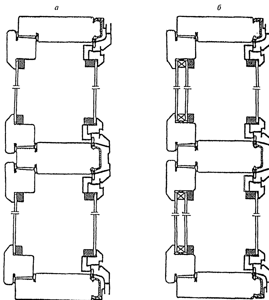
Рисунок 3. Примеры конструктивных решений оконных блоков спаренной (а) и раздельной (б) конструкции с листовым стеклом и стеклопакетом
