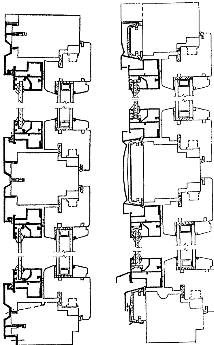
Рисунок 2. Пример конструктивного решения оконного блока спаренной конструкции с листовым стеклом и стеклопакетом
