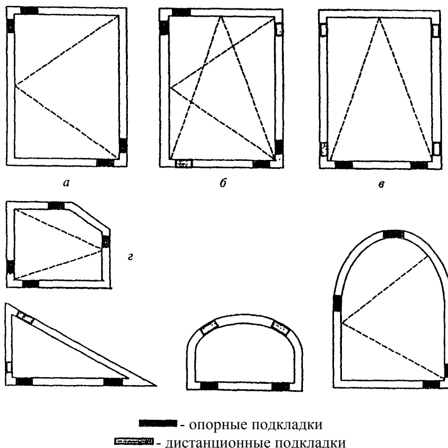
Виды открывания оконных блоков: а - поворотное (распашное); б - поворотно-откидное; в - откидное; г - установка подкладок в фигурных оконных блоках
