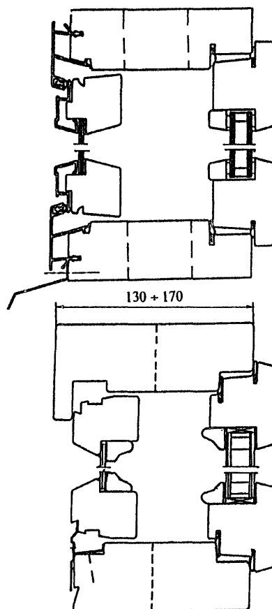
Рисунок 6. Примеры конструктивных решений импостных и безимпостных притворов оконных блоков раздельной конструкции
