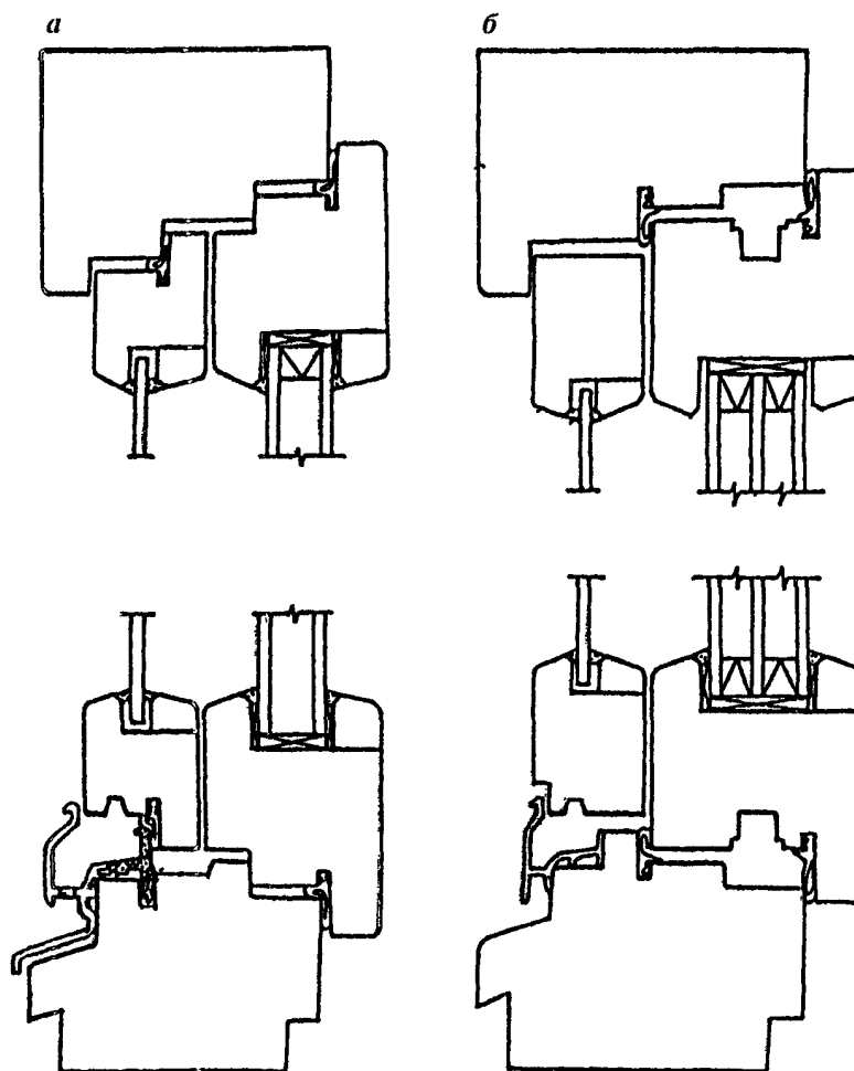
а - вариант конструкции с распашным открыванием створок; внутренняя створка остеклена однокамерным стеклопакетом; с двумя контурами прокладок в наружной и внутренней створках; с алюминиевым дождезащитным профилем с термовставкой; б - вариант конструкции с поворотно-откидным открыванием створок; внутренняя створка остеклена двухкамерным
