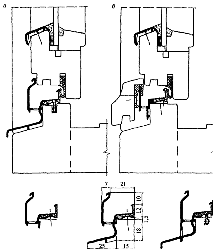
Рисунок 11. Примеры горизонтального (а) и вертикального (б) сечений оконного блока спаренной конструкции с алюминиевыми облицовочными профилями
