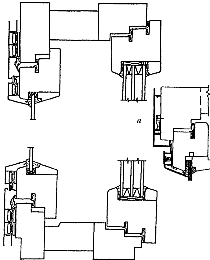
а - вариант конструкции облицовки
