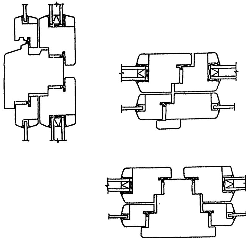
Рисунок 3. Примеры конструктивных решений импостных и безимпостных притворов оконных блоков спаренной конструкции (вариант распашного открывания)
