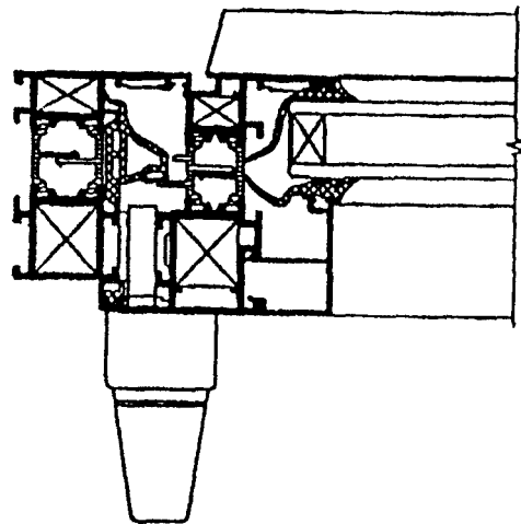
Рисунок 3. Вариант конструктивного решения узлов притвора оконного блока с поворотно-откидным открыванием внутрь помещения
