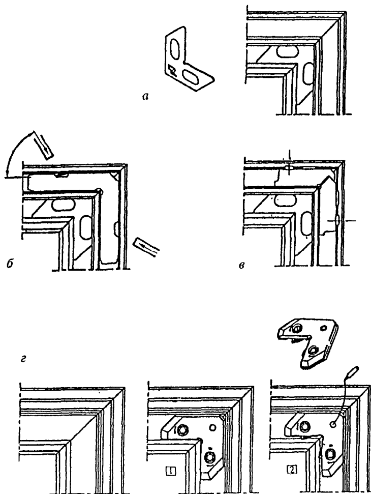
а - соединительный уголок; б - соединение опрессовкой крепёжного уголка; в - соединение крепёжным уголком с дополнительной фиксацией винтами; г - соединение уголком с эксцентриковым зажимом
