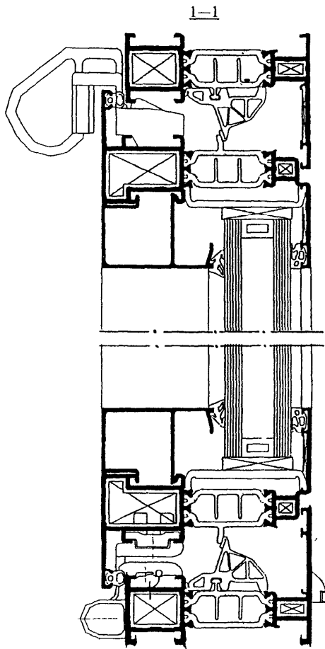
Рисунок 2. Пример конструктивного решения оконного блока с откидным открыванием створки внутрь помещения
