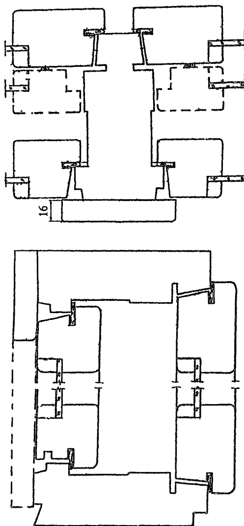
Рисунок 7. Пример раздельной конструкции оконного блока с двойным остеклением (бруски коробки имеют универсальный профиль, что позволяет устанавливать дополнительную створку и преобразовывать конструкцию в раздельно-спаренную)
