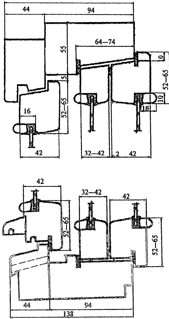
Рисунок 5. Примеры конструктивных решений оконных блоков раздельно-спаренной конструкции
