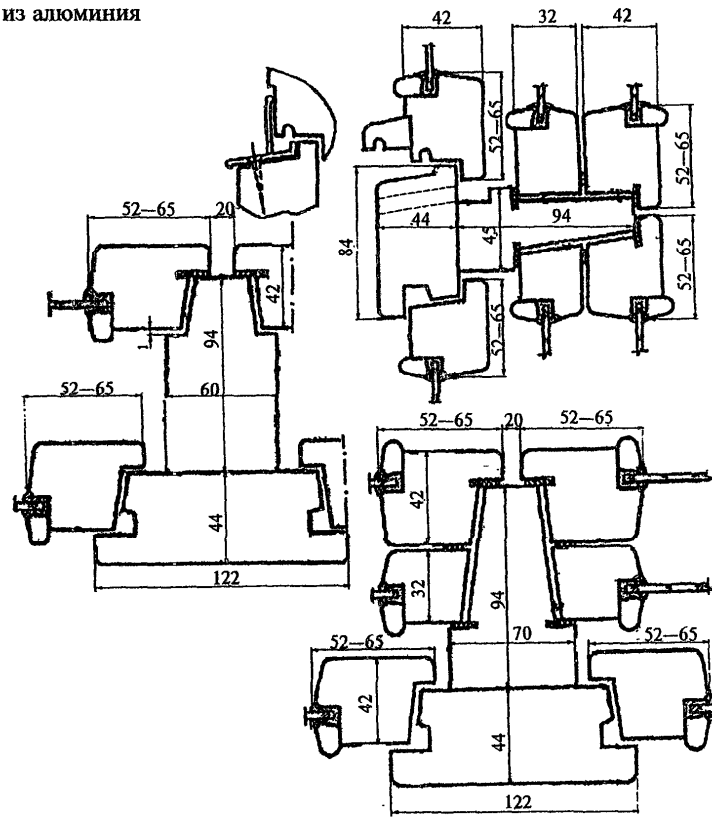
Рисунок 6. Примеры конструктивных решений узлов импостных притворов оконных блоков раздельной и раздельно-спаренной конструкции
