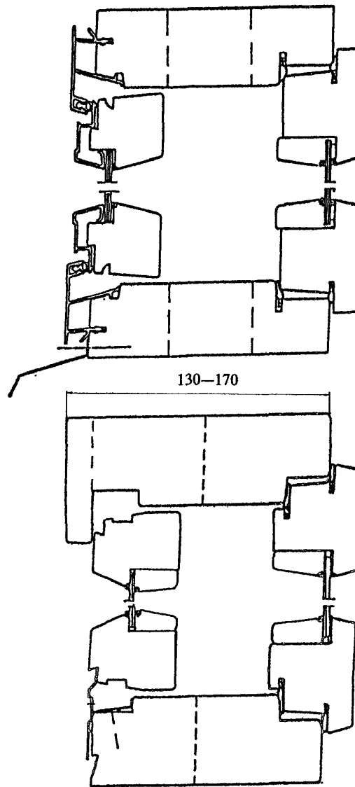
Рисунок 9. Примеры конструктивных решений оконных блоков раздельной конструкции с безнаплавной наружной створкой (основной и нижний притворы)
