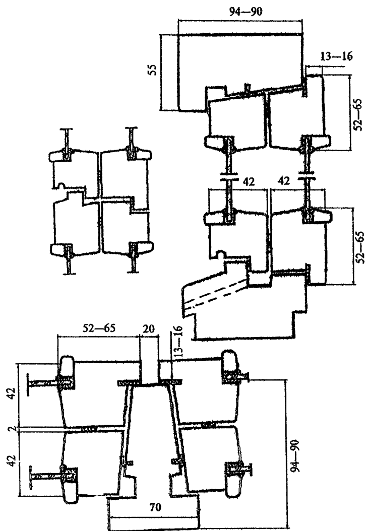
Рисунок 3. Примеры конструктивных решений оконных блоков спаренной конструкции (с распашным открыванием створок, двумя рядами уплотняющих прокладок наплав толщиной 16 мм - под ввертную петлю)
