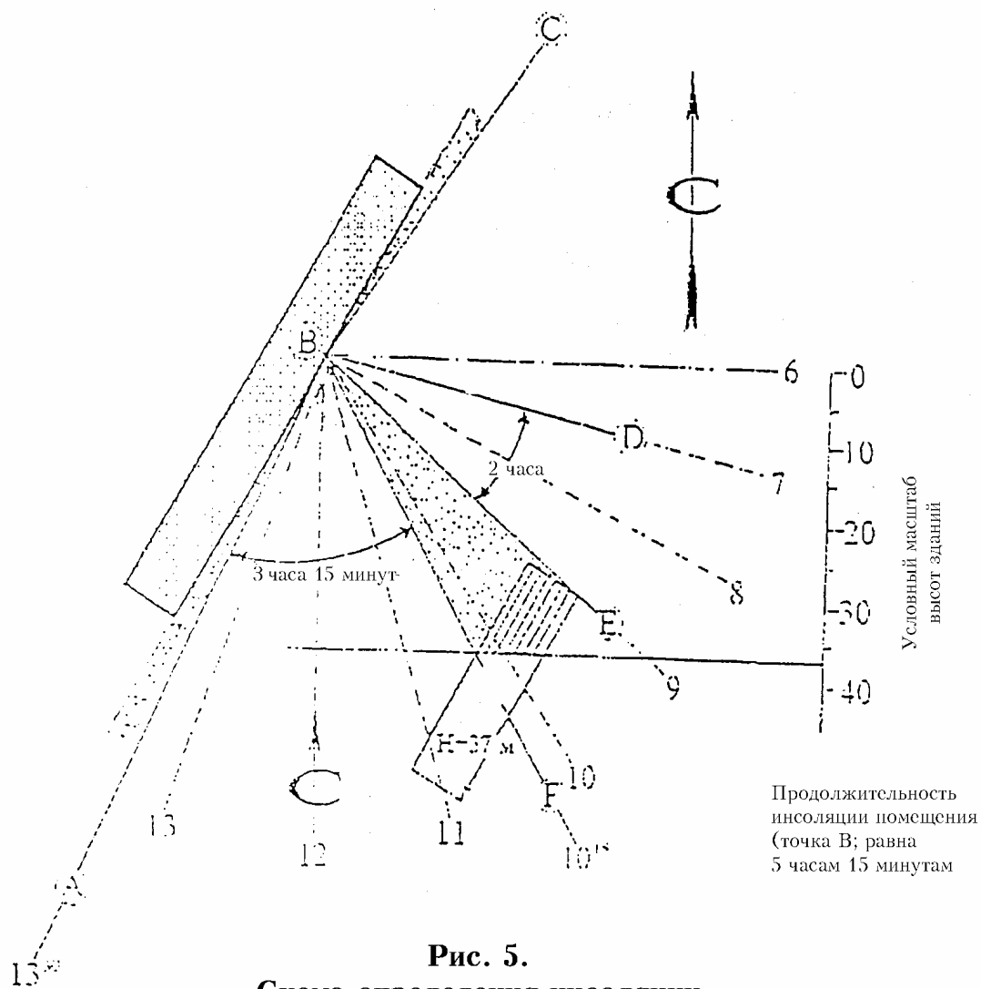
"Рис. 5. Схема определения инсоляции"
