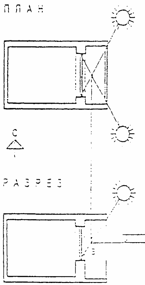
Рис. 3. Схема определения расчетной точки для окна с лоджией.
