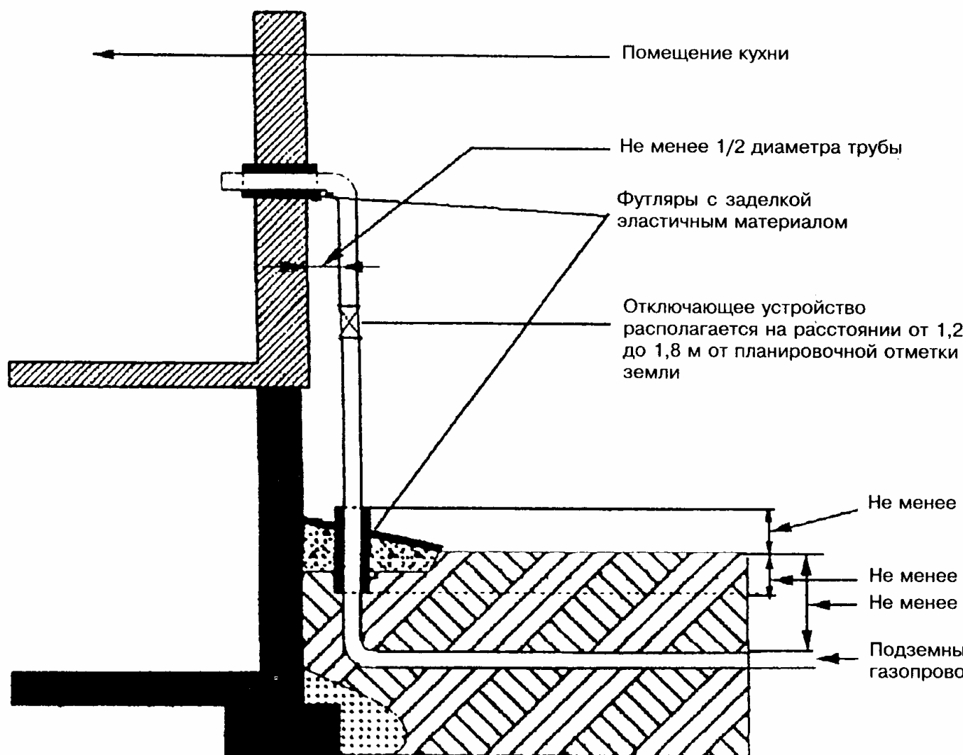
Рисунок 9.1 — Газовый ввод
