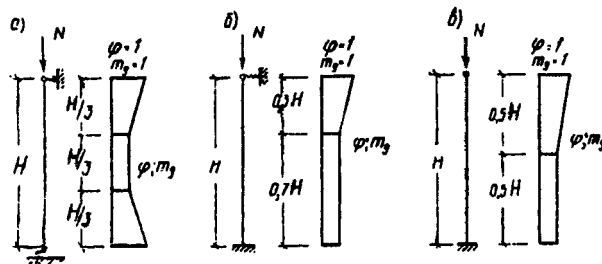
Рис. 4. Коэффициенты \varphi и m_g по высоте сжатых стен и столбов
