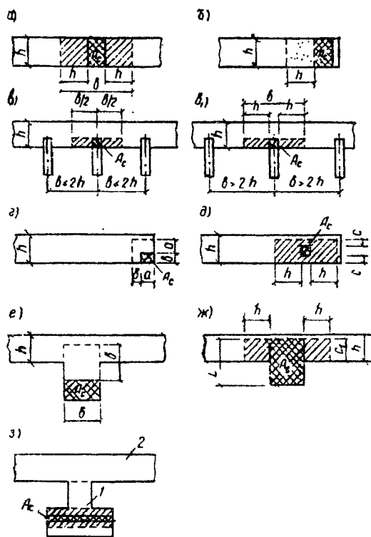
Рис. 9. Определение расчетных площадей
