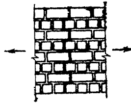
Рис. 1. Растяжение кладки по неперевязанному сечению
