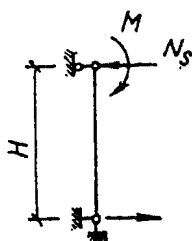
Рис. 12. Определение усилия в анкере от изгибающего момента в уровне перекрытия
