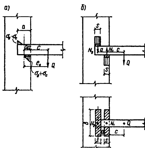
Рис. 14. Расчетные схемы заделки консольных балок
