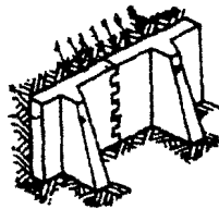
Рис. 3. Растяжение кладки при изгибе по перевязанному сечению
