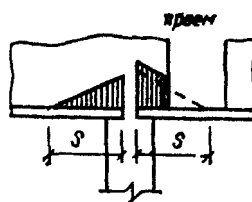
Рис. 16. Эпюра распределения давления в кладке висячих стен при наличии проема
