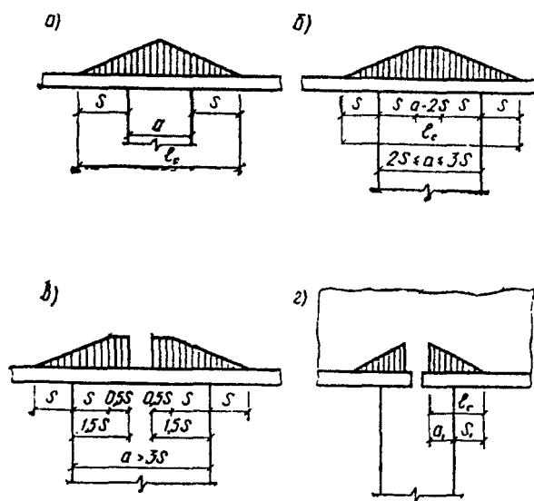
Рис. 15. Распределение давления в кладке над опорами висячих стен
