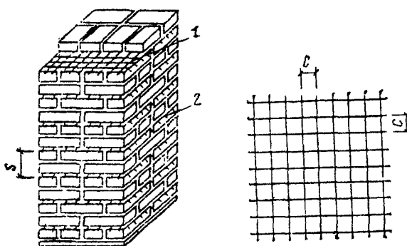
Рис. 10. Поперечное (сетчатое) армирование каменных конструкций
