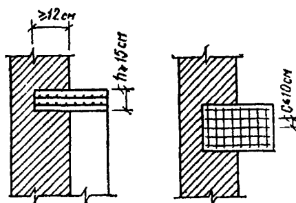
Рис. 13. Железобетонные распределительные плиты
